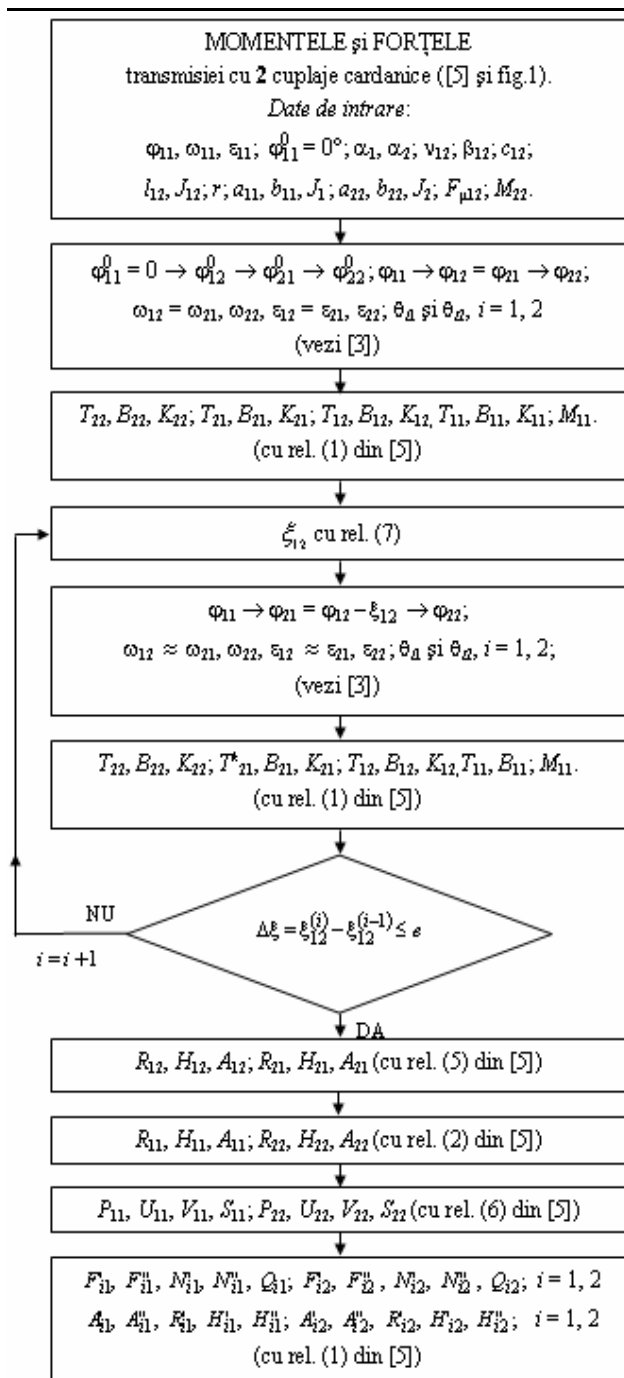
Fig. 2. Organigrama algoritmului de modelare modulară al unei transmisiuni bicardanice, în premisa că arborele intermediar este elastic
