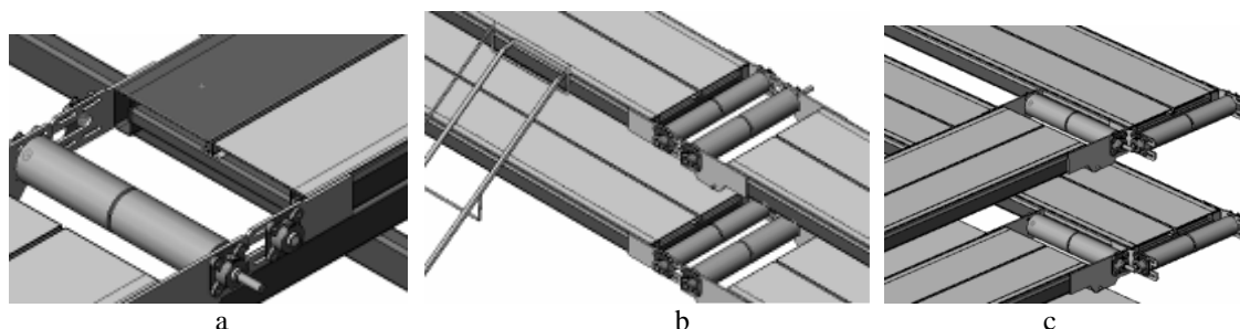
Figura 11 a,b,c. Ansamblul suport al benzilor transportoare Figure 11 a,b,c. The support rubber bands assembly
